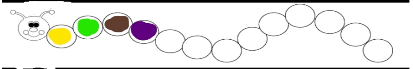
Μοτίβο ΑΒΒΑ
