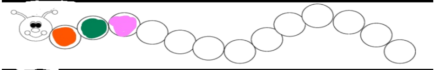
Μοτίβο ΑΒΓΔ
