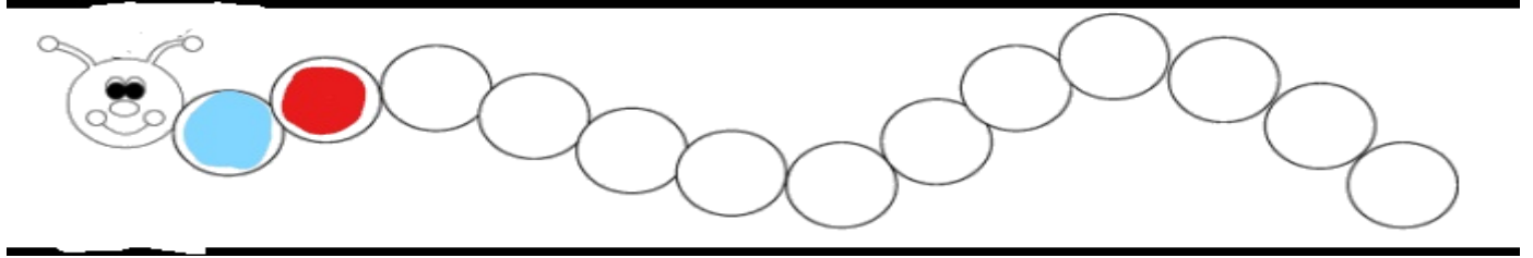
Μοτίβο ΑΒΓ
