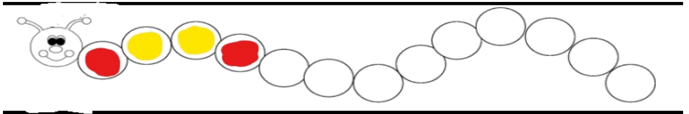
Μοτίβο ΑΑΒΑΑ
