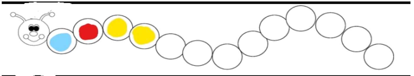
Μοτίβο ΑΒΓΓ
